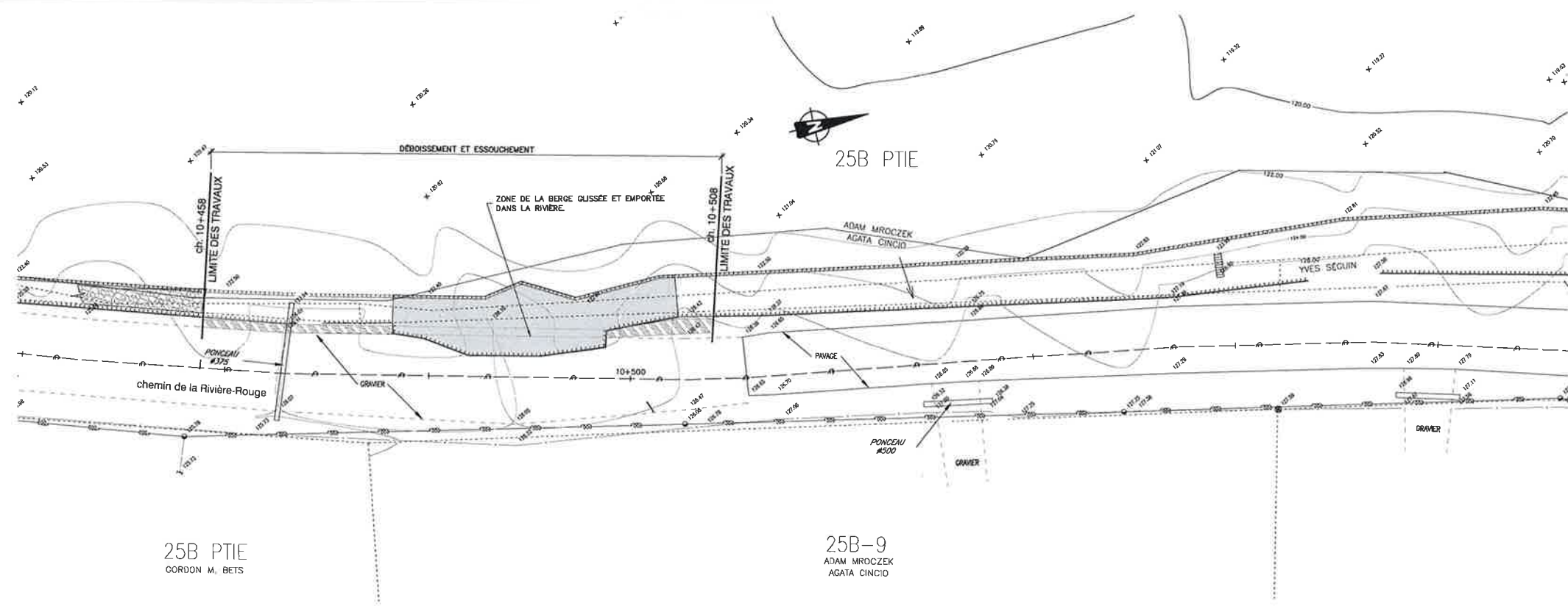
VUE EN PLAN EXISTANT Echelle: 1=250
