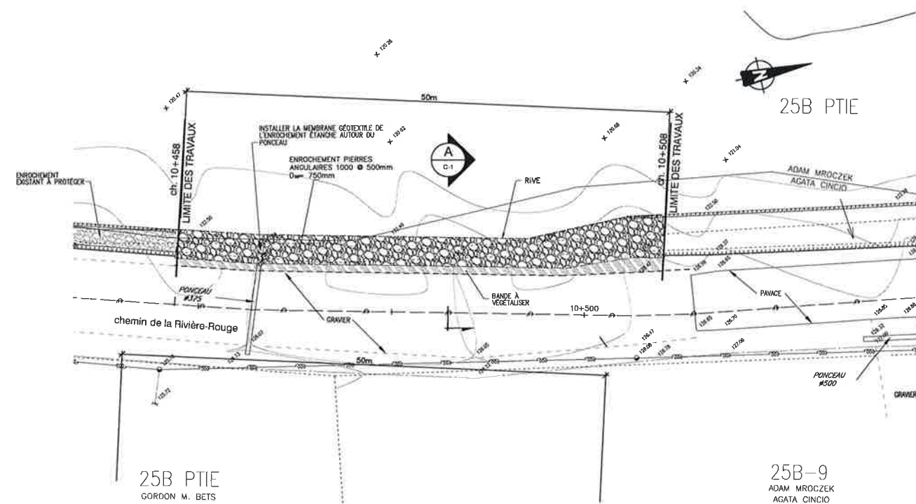
VUE EN PLAN AMÉNAGEMENT PROPOSÉ Echelle: 1=250
