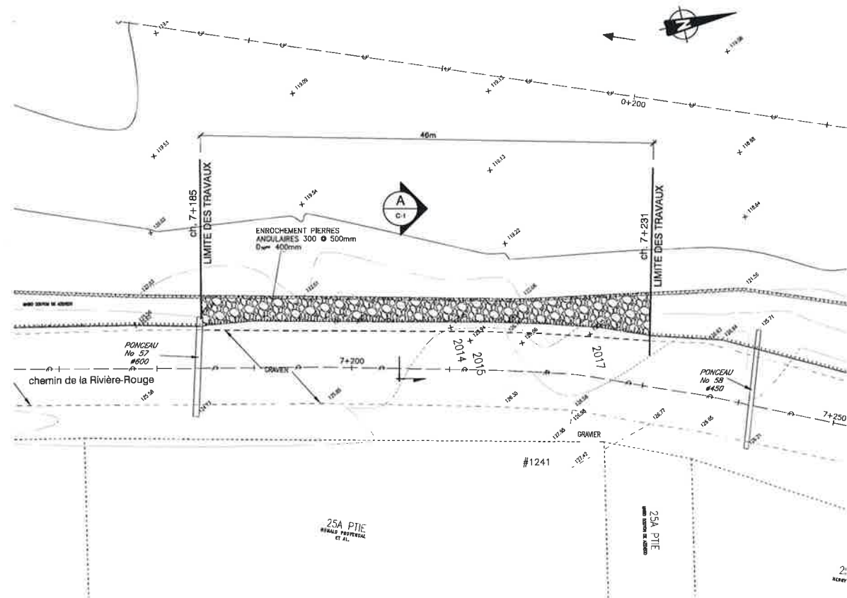
VUE EN PLAN AMÉNAGEMENT PROPOSÉ ÉCHELLE: 1=250
